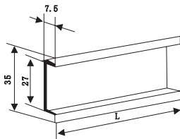
图3 安装轨尺寸图
