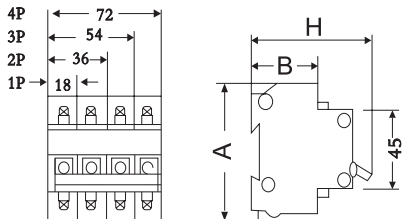
图2 外形尺寸图
