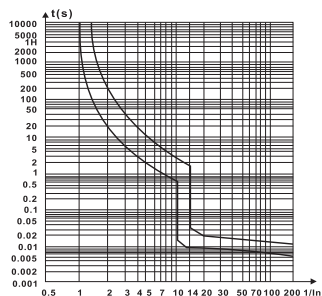
D型特性曲线
