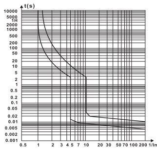
C型特性曲线
